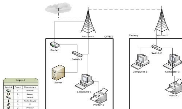
Gambar 3.4 Rancangan Struktur Jaringan Komputer
